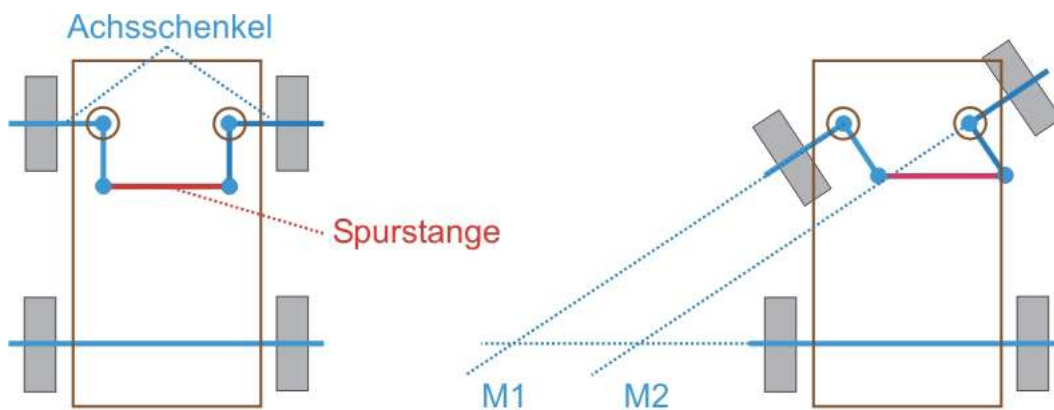
Parallelogrammlenkung
