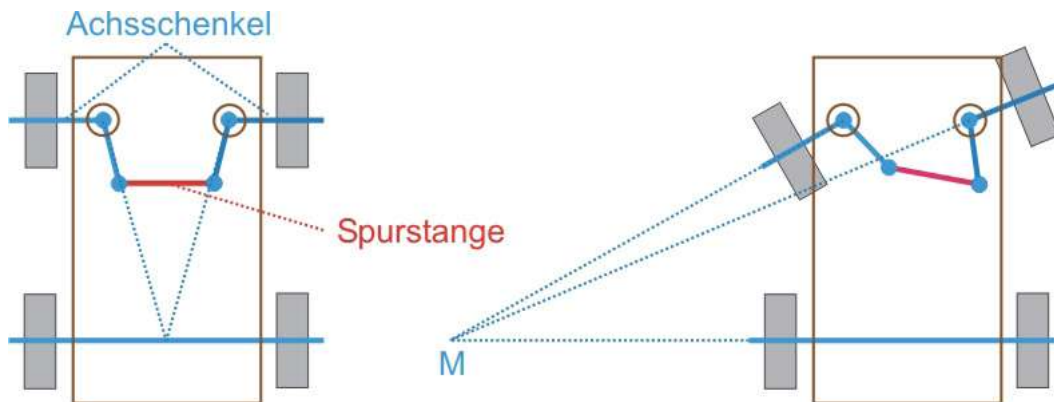
Trapezlenkung
